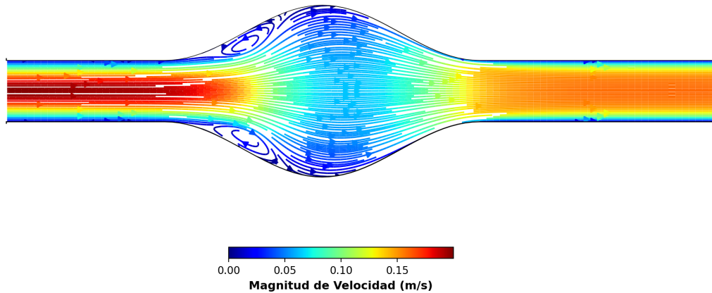
Figura 4: Líneas de corriente para un caudal de 0,42 \cdot 10^{-4} m 3 /s, número de Reynolds de 812 y velocidad máxima de 0,2 m/s.
